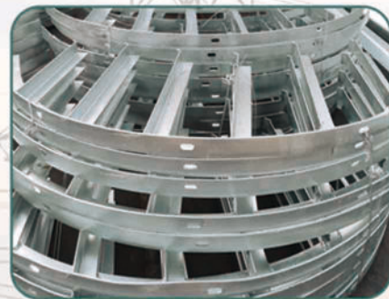
电缆支架 Cable support
